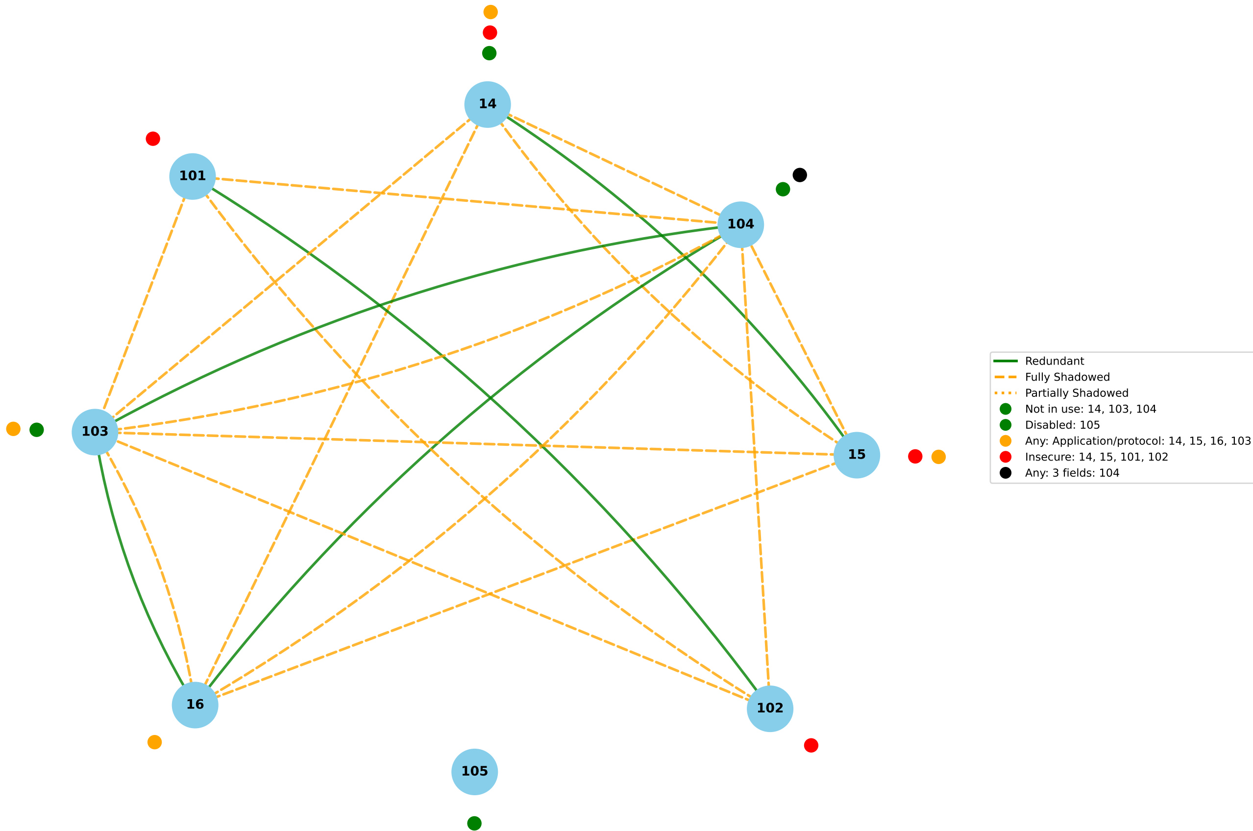
Grafo de Conflictos de Reglas de Firewall
